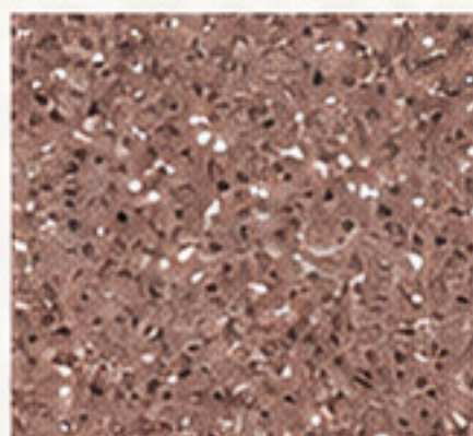
203 IDV- TZ
