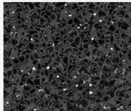
851 IDV- TZ
