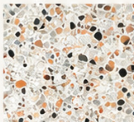
924 IDV- TZ
