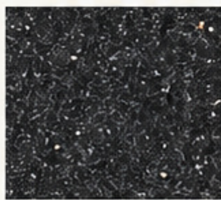
809 IDV- TZ
