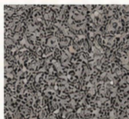
855 IDV- TZ
