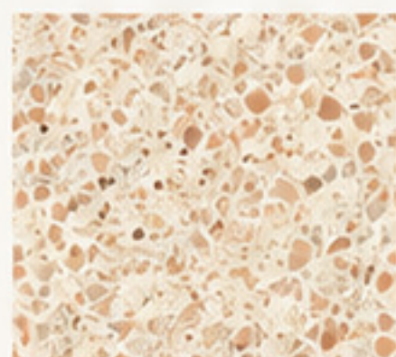
901 IDV- TZ
