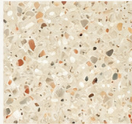
700 IDV- TZ
