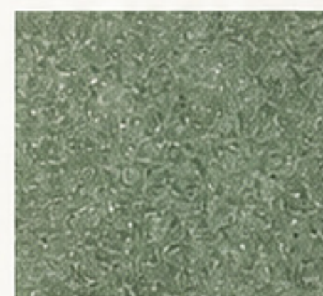
288 IDV- TZ
