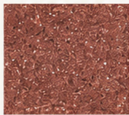
252 IDV- TZ
