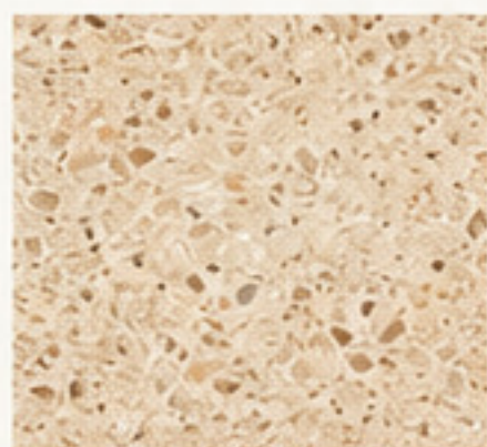
644 IDV- TZ
