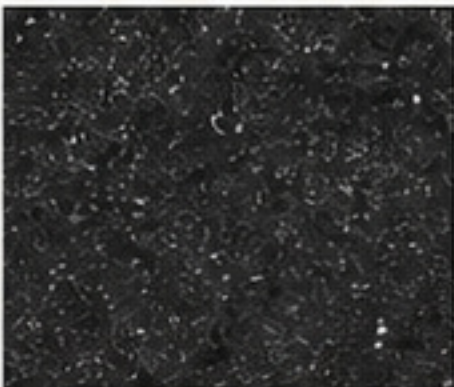
810 IDV- TZ
