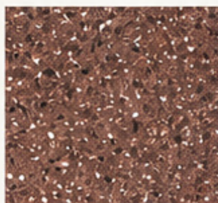
255 IDV- TZ
