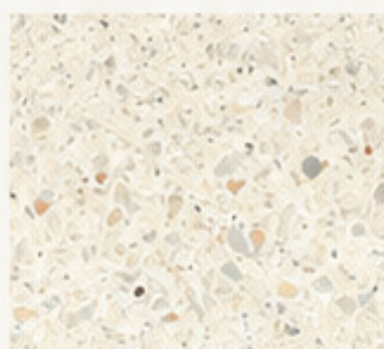
301 IDV- TZ
