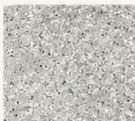
222 IDV- TZ
