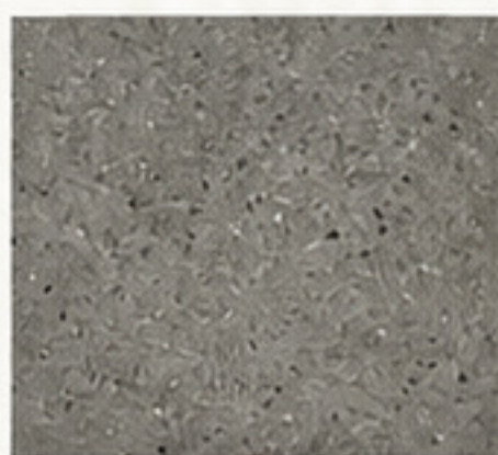
785 IDV- TZ
