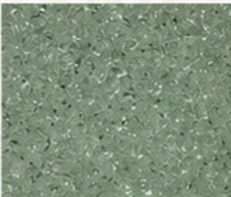
282 IDV- TZ
