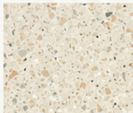
302 IDV- TZ
