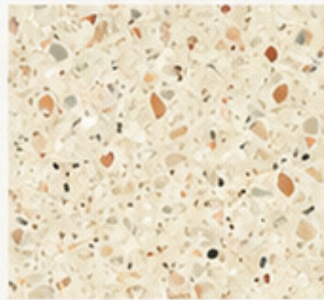
371 IDV- TZ
