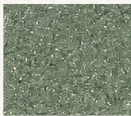
288 IDV- TZ
