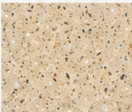
620 IDV- TZ
