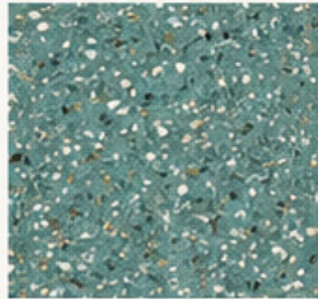
244 IDV- TZ
