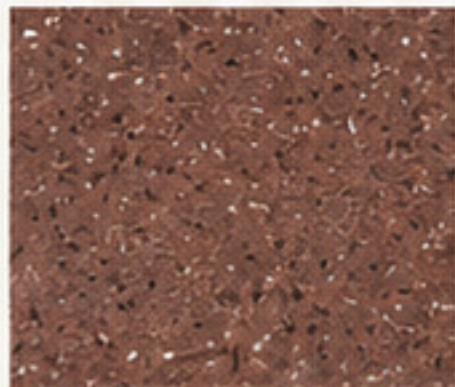
251 IDV- TZ
