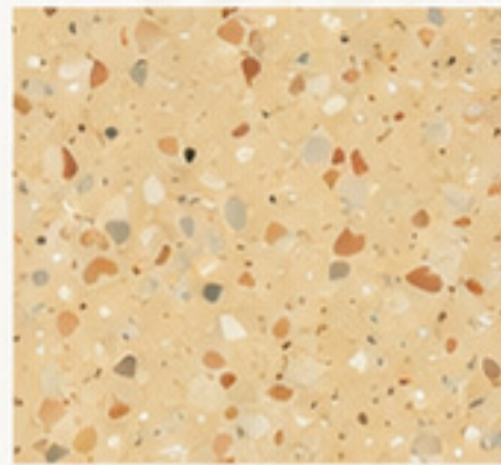
606 IDV- TZ
