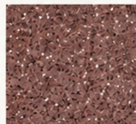
203 IDV- TZ
