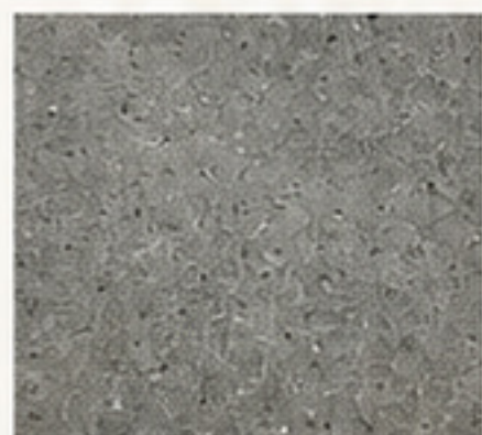
785 IDV- TZ
